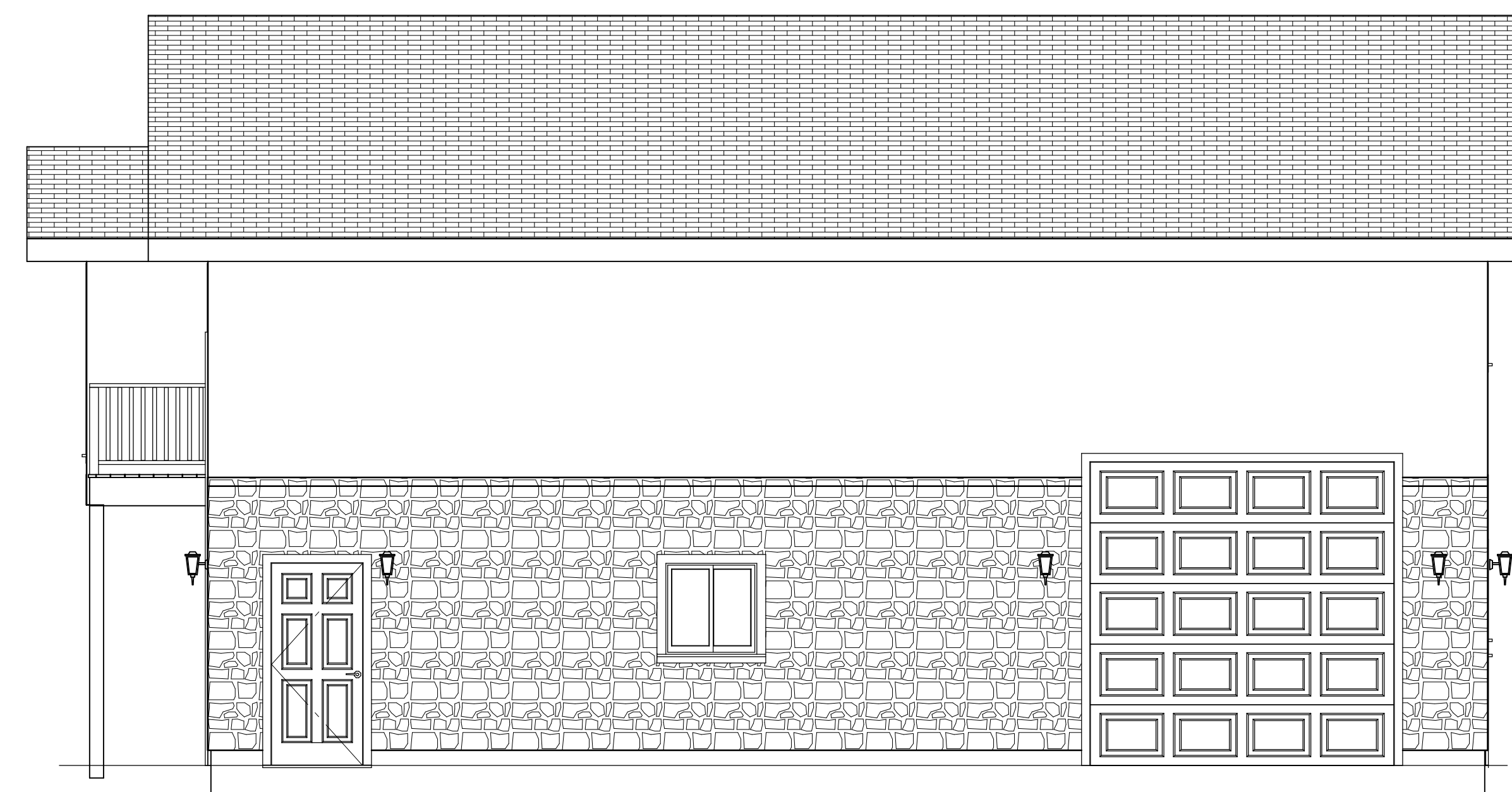
RIGHT ELEVATION SCALE: 1/4" = 1'
