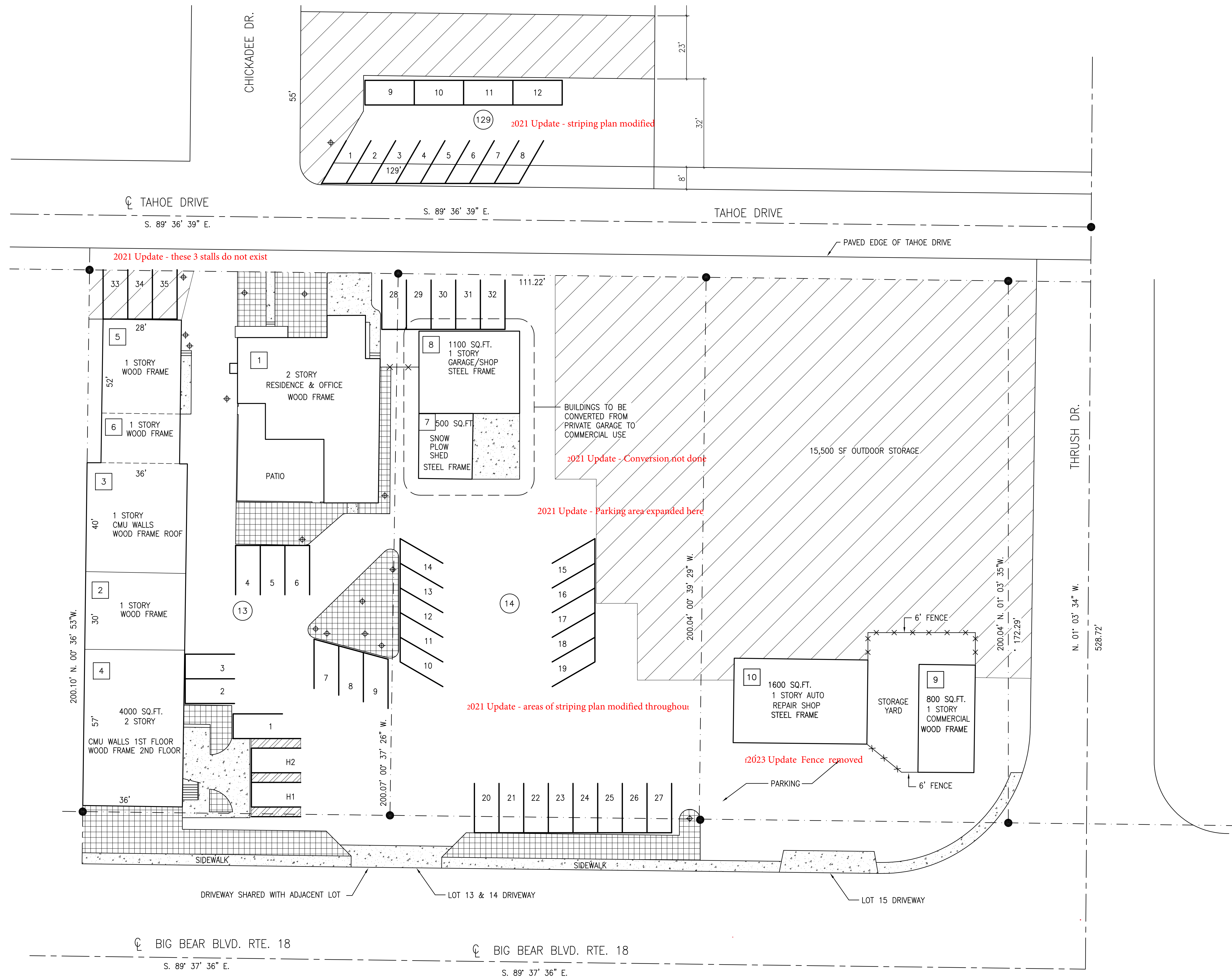
1 SITE PLAN 1/16"=1'-0"
