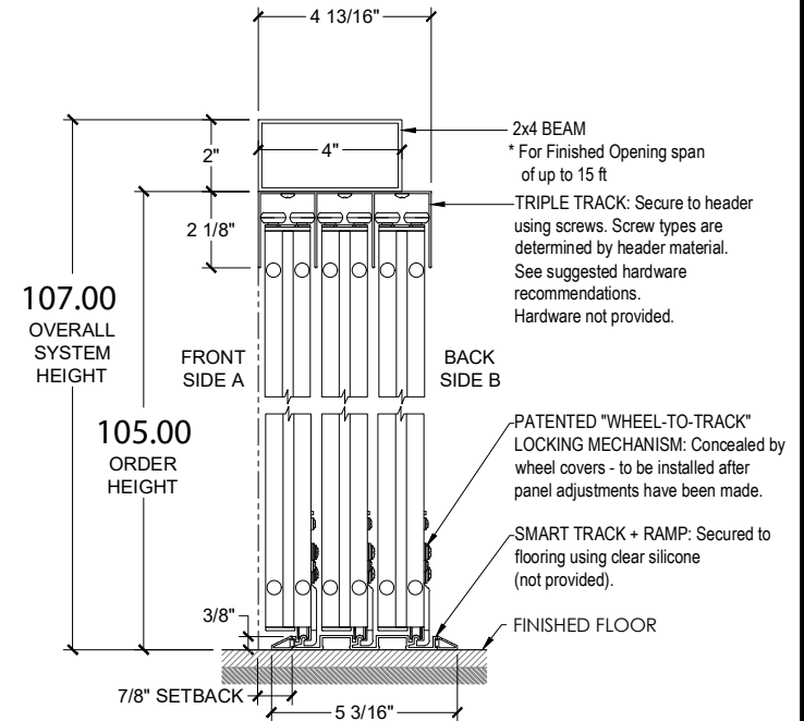
S1 - SECTION 1: Scale: None
